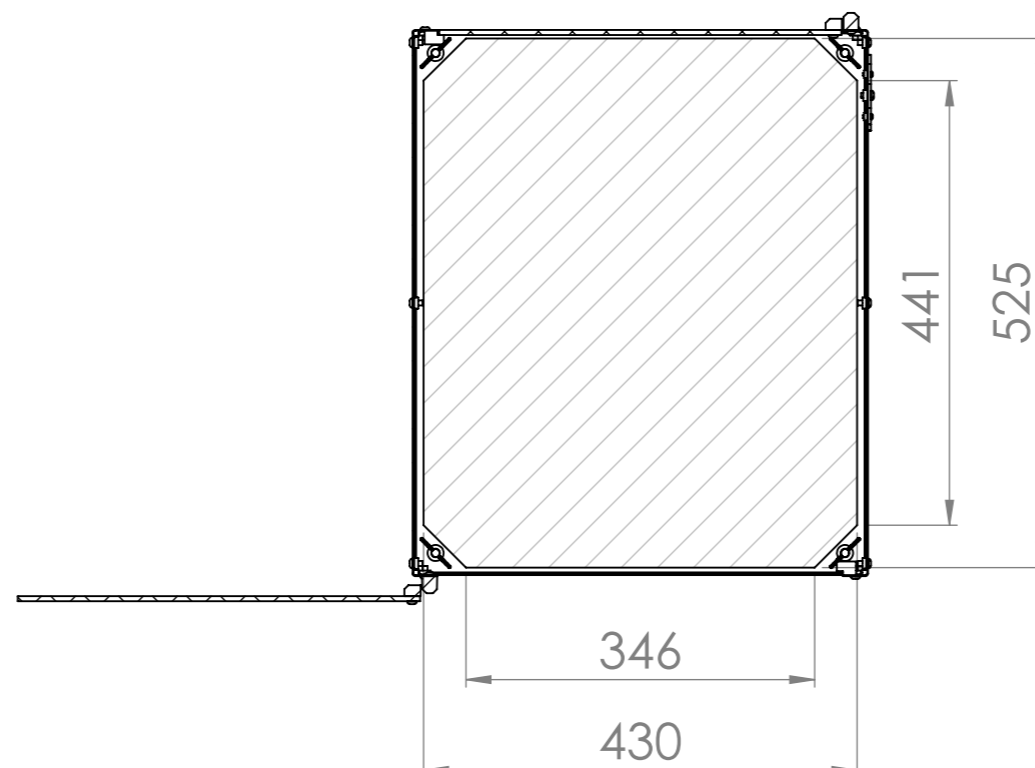
SECTION A-A
